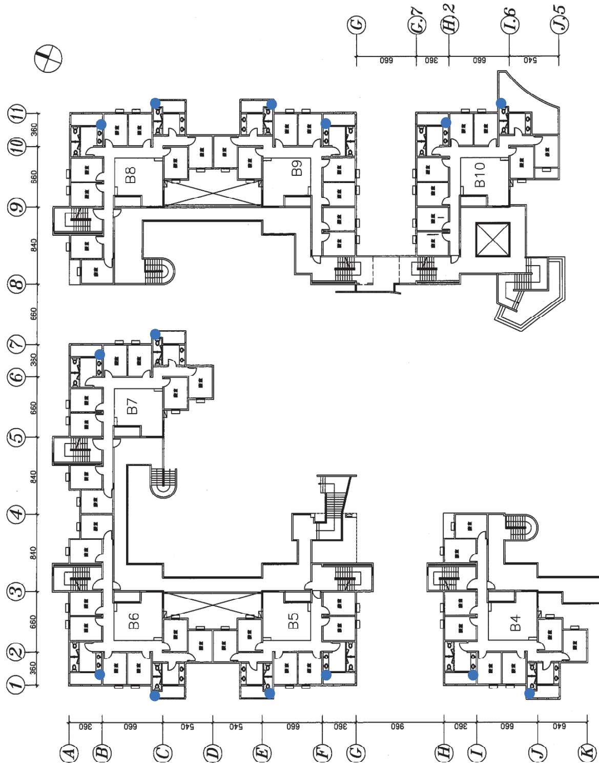
嶺雲二廿貳層寢室平面圖
