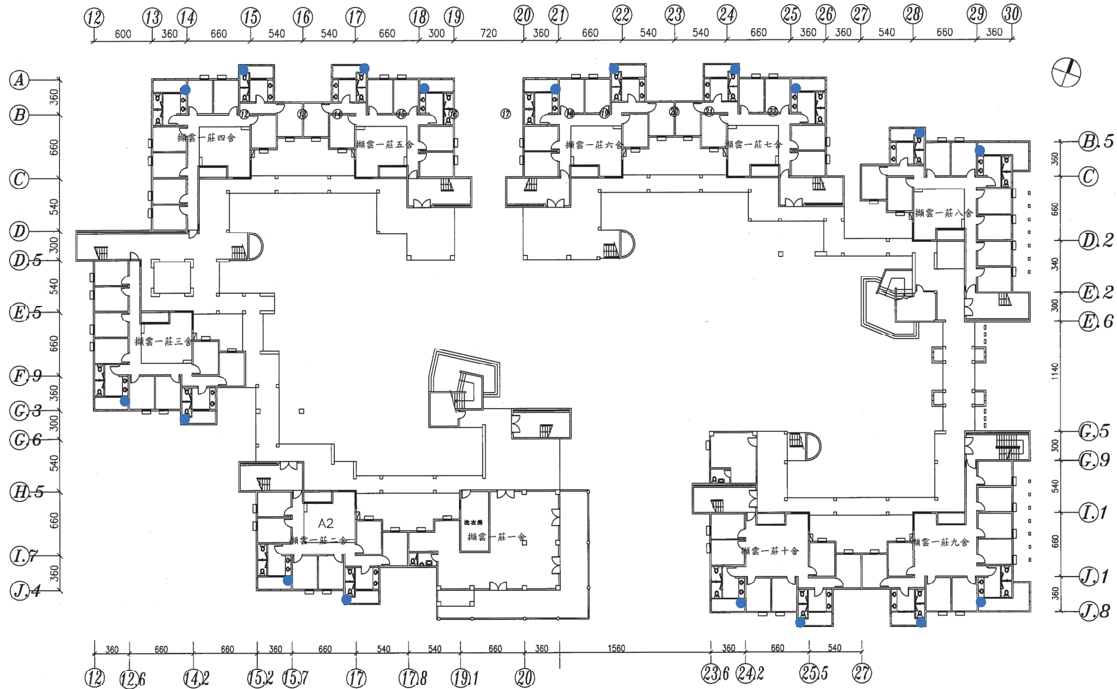
擷雲一莊壹樓各寢室平面圖
