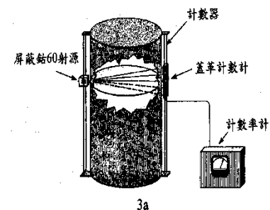
液位计 Level meter
