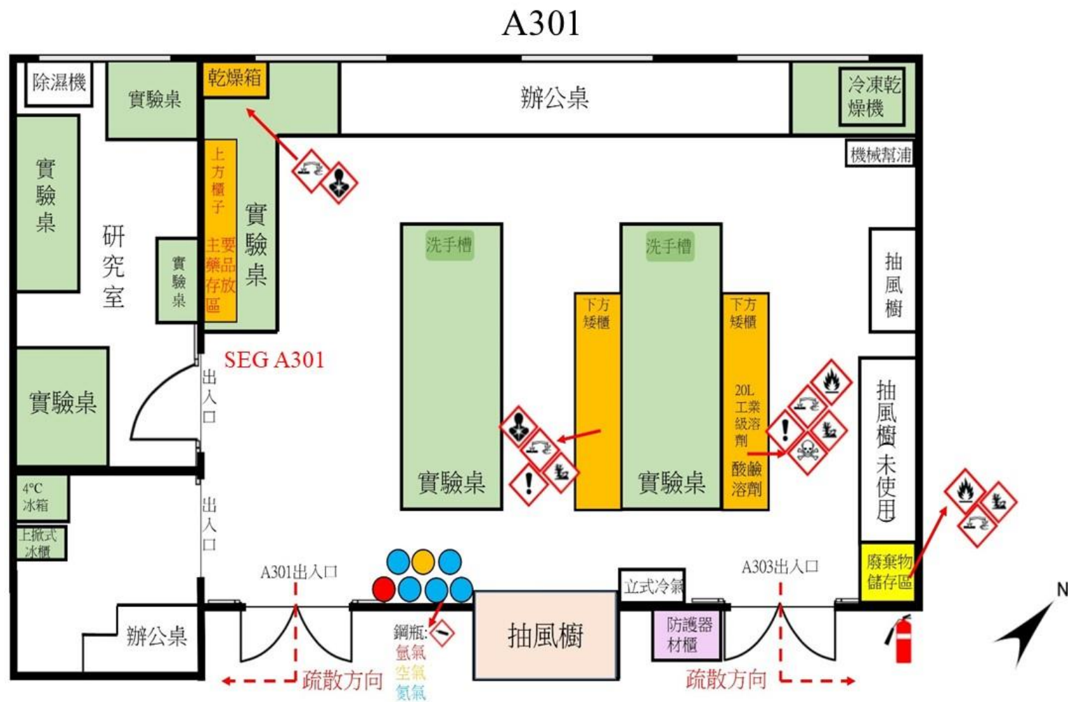
圖二-1、工作場所配置圖
